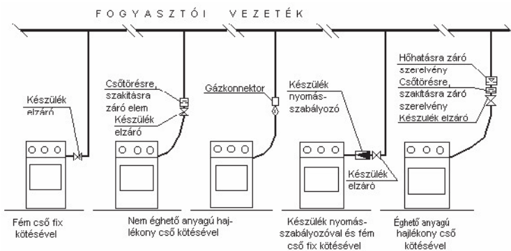
Gömbcsap hőhatásra záró biztonsági szeleppel / Ball valve with thermal safety device
