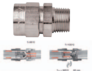
Hőhatásra záró szelep • Kioldási hőmérséklet: 95 – 100 °C • Lezárási idő max.: 60 sec. • Maximális nyomás: 0.5 MPa (5 bar) MOP 5 • Termikus terhelhetőség: 925 °C (60 min.-ig) • Környezeti hőmérséklet max.: 80 °C • Anyag: rozsdamentes acél • Csomagolási egység: 10 db/ doboz
