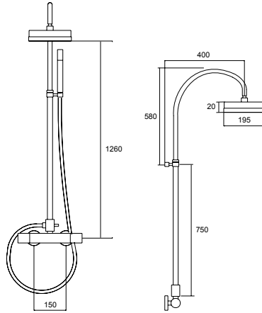
Grupo de ducha termostático redondo con kit de ducha y barra Rounded thermostatic shower mixer with shower kit and bar
